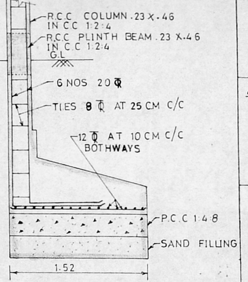
COLUMN L' TYPE FOUNDATION
